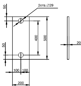
Опорная плита 500x200
