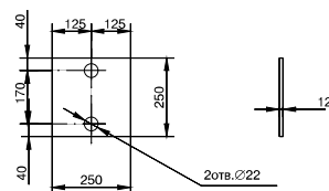
Опорная плита 250x250
