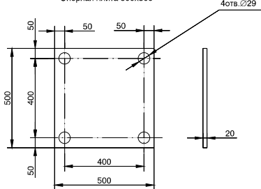
Опорная плита 500x500
