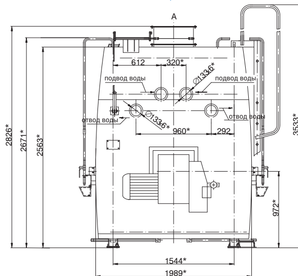
КВ-ГМ-4,65-115Н
