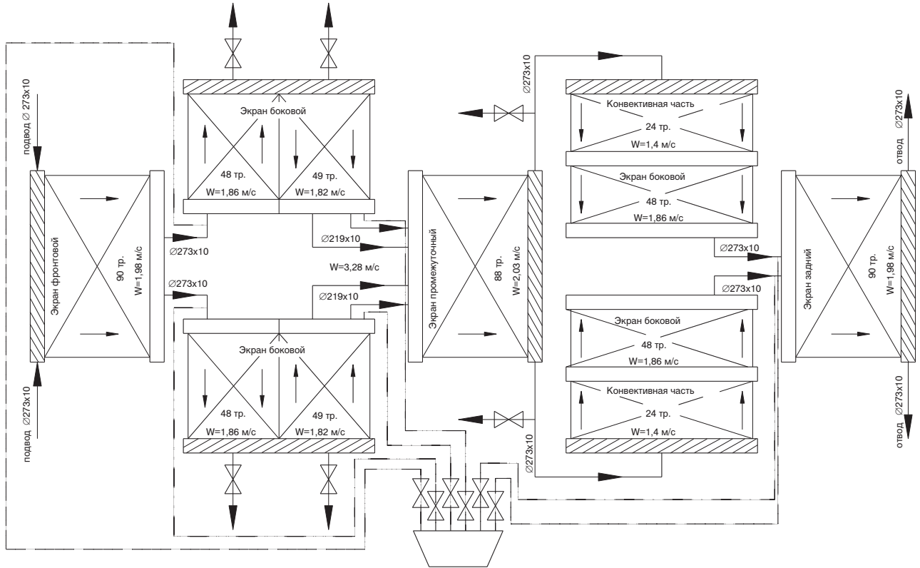
Схема гидравлическая принципиальная котла КВ-ГМ-139,6-150
