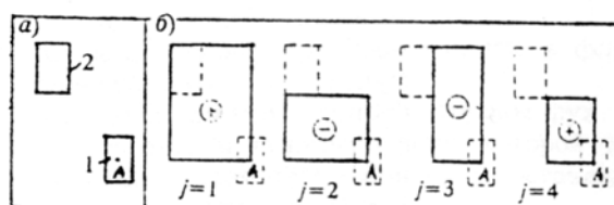
рис.2. Схема к определению дополнительных вертикальных напряжений \sigma_{p,\alpha} в основании рассчитываемого фундамента с учетом влияния соседнего фундамента методом угловых точек
