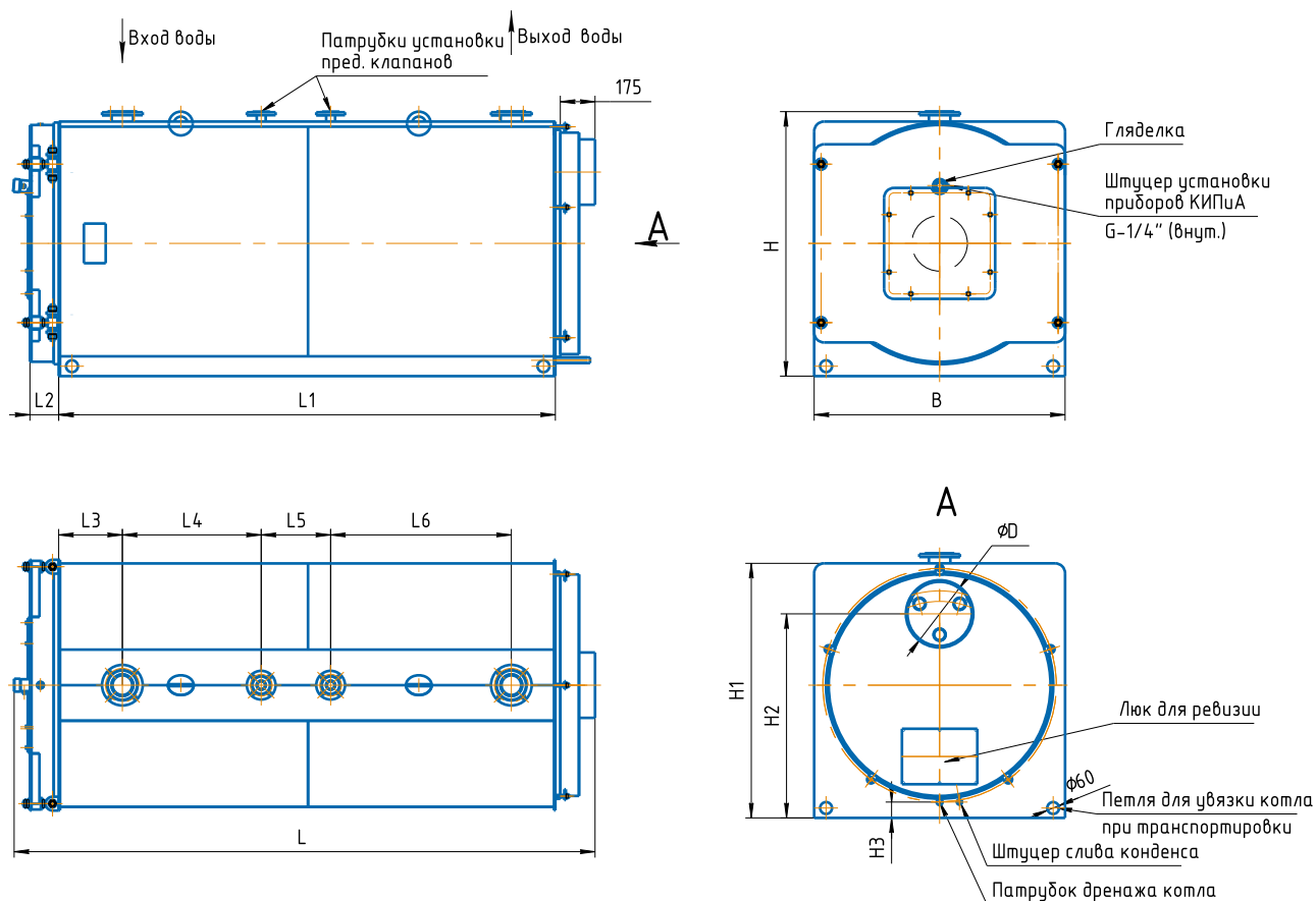
Рис.1 Общий вид котла.
